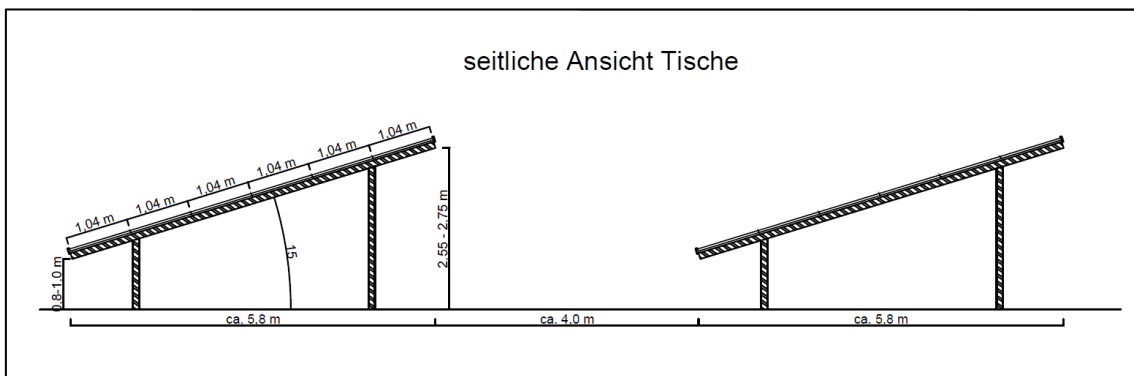
Abb.: Abmessung und Anordnung der Solarmodule (Technische Planung AHS Solar)
